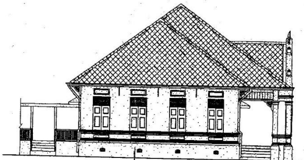
รูปด้าน ทิศใต้ มาตราส่วน 1:100
