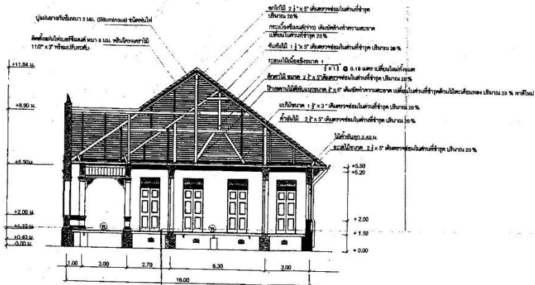
รูปตัด ② - ② มาตราส่วน 1:100
